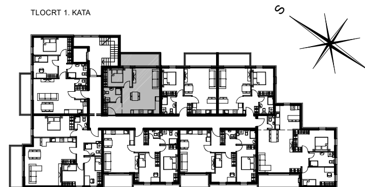
TLOCRT 1. KATA
