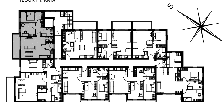
TLOCRT 1. KATA
