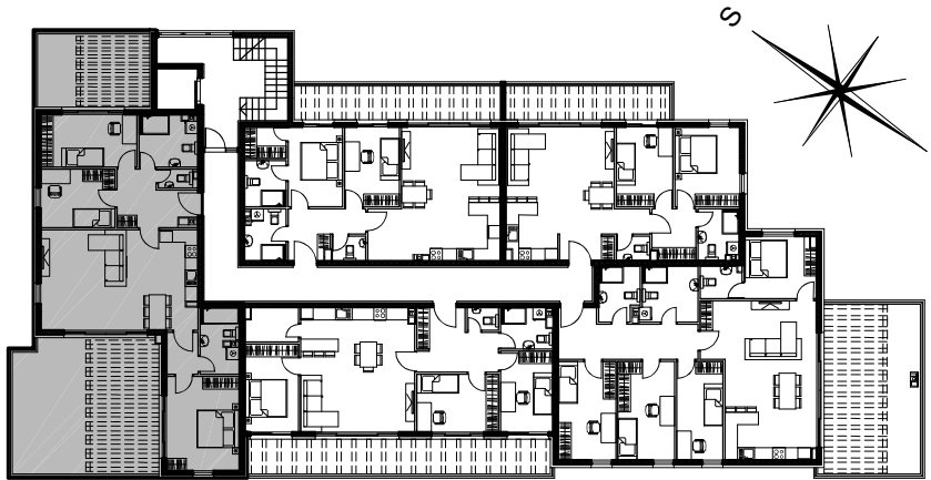
TLOCRT 4. KATA
