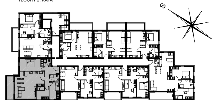
TLOCRT 2. KATA
