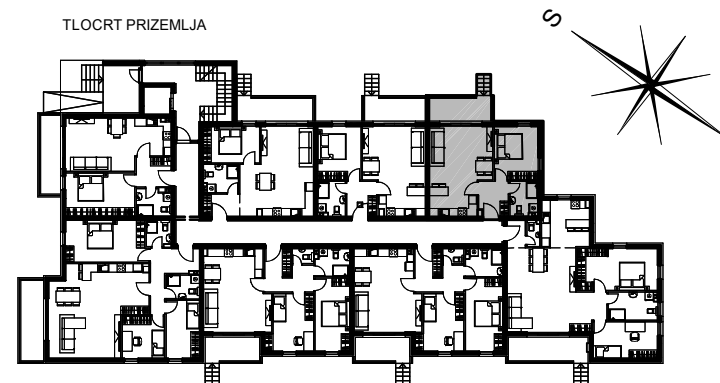
TLOCRT PRIZEMLJA
